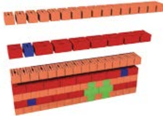
Kreuzverband
