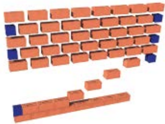
Läuferverband
